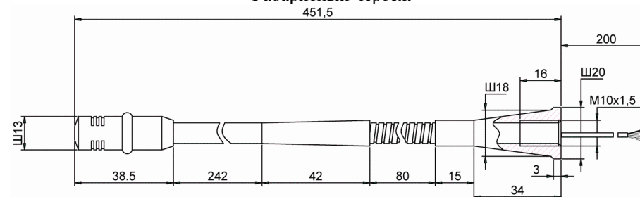
Габаритный чертеж
